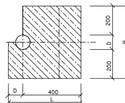
BET. BLOK /B 135/ FIXUJE KOLENÁ
