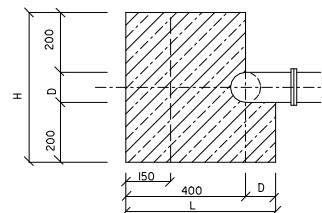
BET. BLOK /B 135/ FIXUJE ODBOČKY
