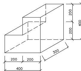
BET. BLOK /B 135/ FIXUJE TVAROVKU "PP"
