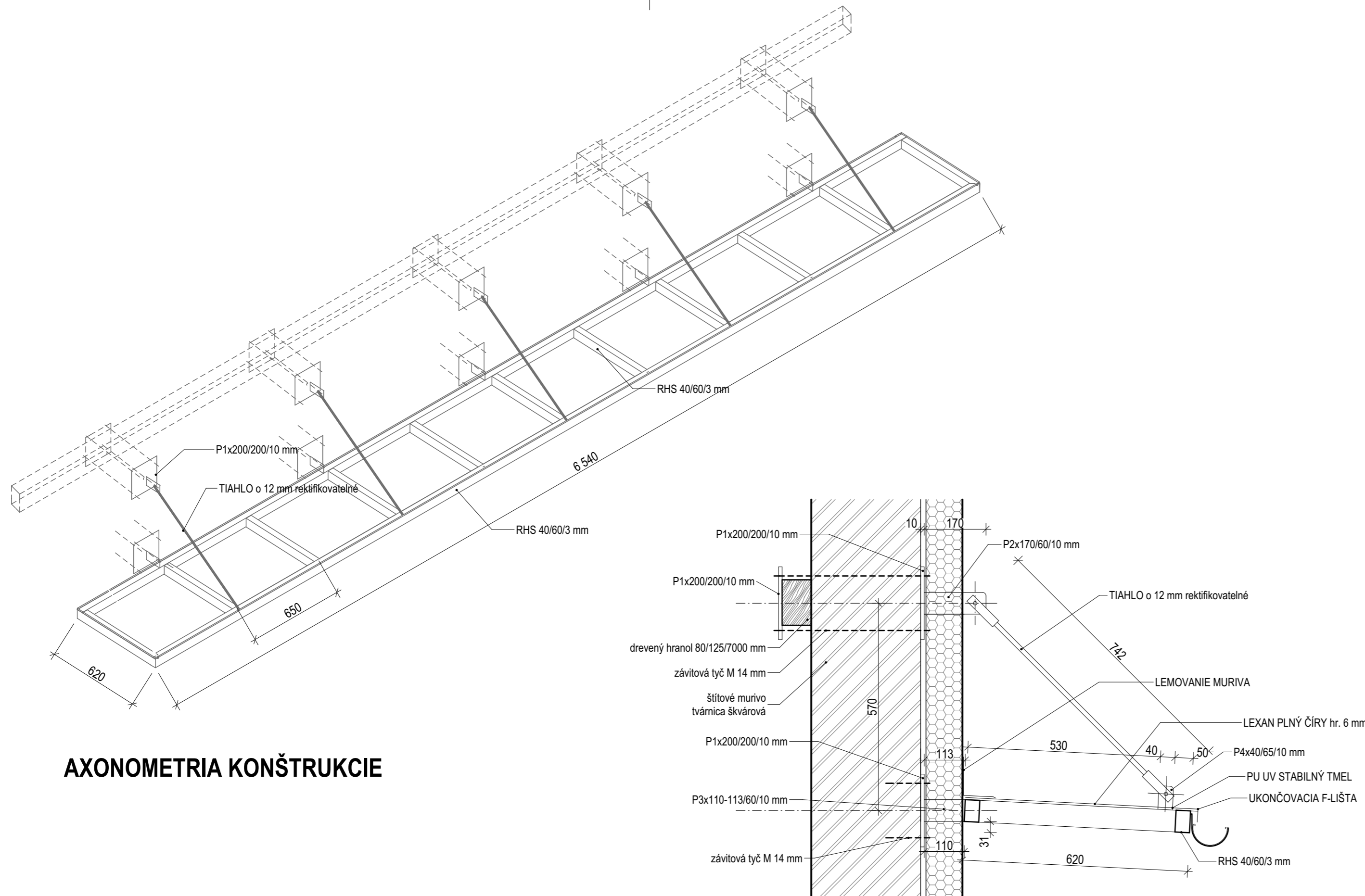
DETAIL UKOTVENIA
