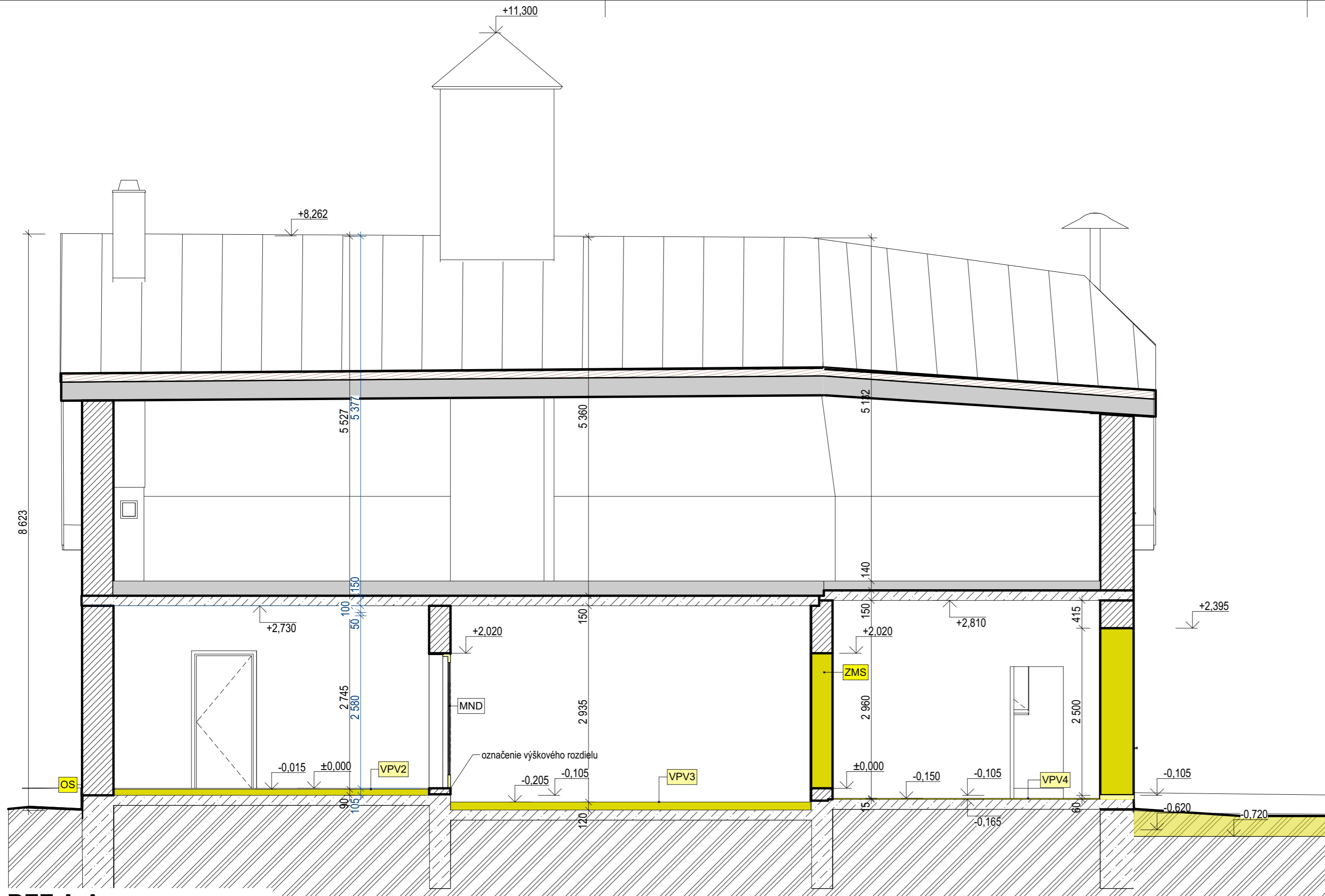
REZ A-A BÚRACIE PRÁCE M1:50
